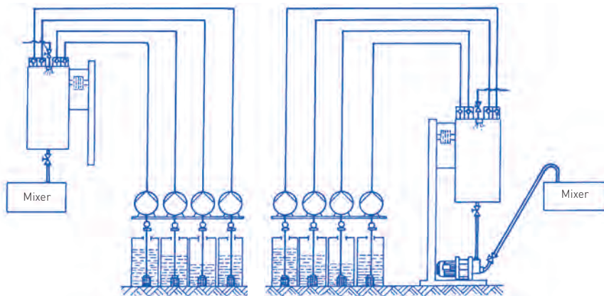
▲ Весы с четырьмя наполняющими насосами, разгрузка самотеком в смеситель
