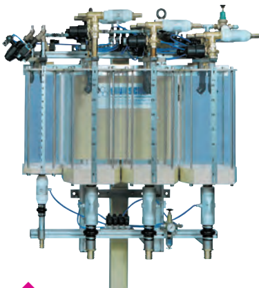
▲ KFW 12,5/25/25/25 Весы с 4 цилиндрами, 1 на 15 л для добавок и 3 по 30 л для суспензий
